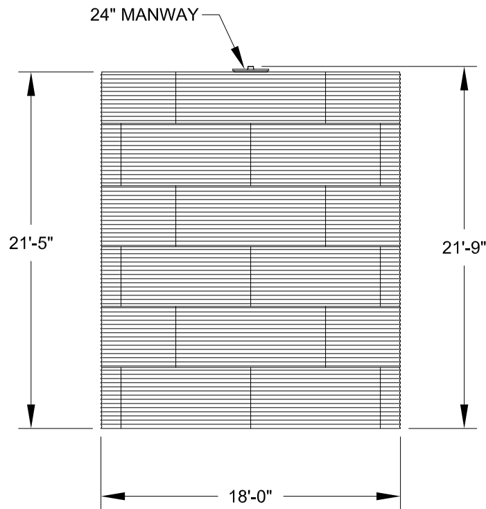
ELEVATION
