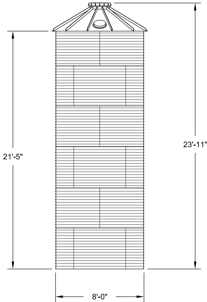
ELEVATION
