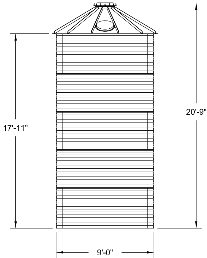
ELEVATION
