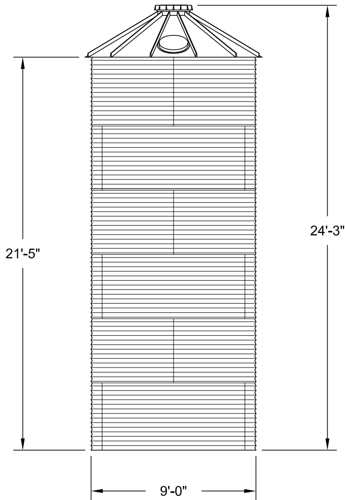
ELEVATION
